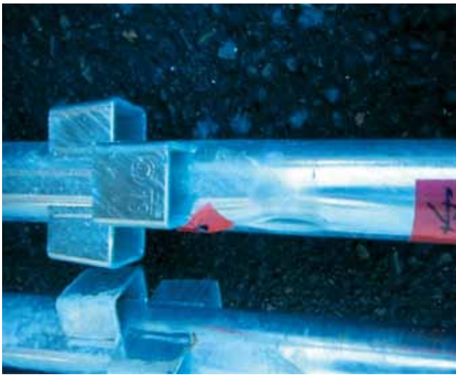
A-2 パイプ部分の曲がり、変形、へこみ
